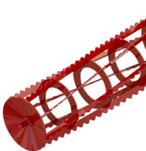
Rouleau crénelé Ø 280 mm
